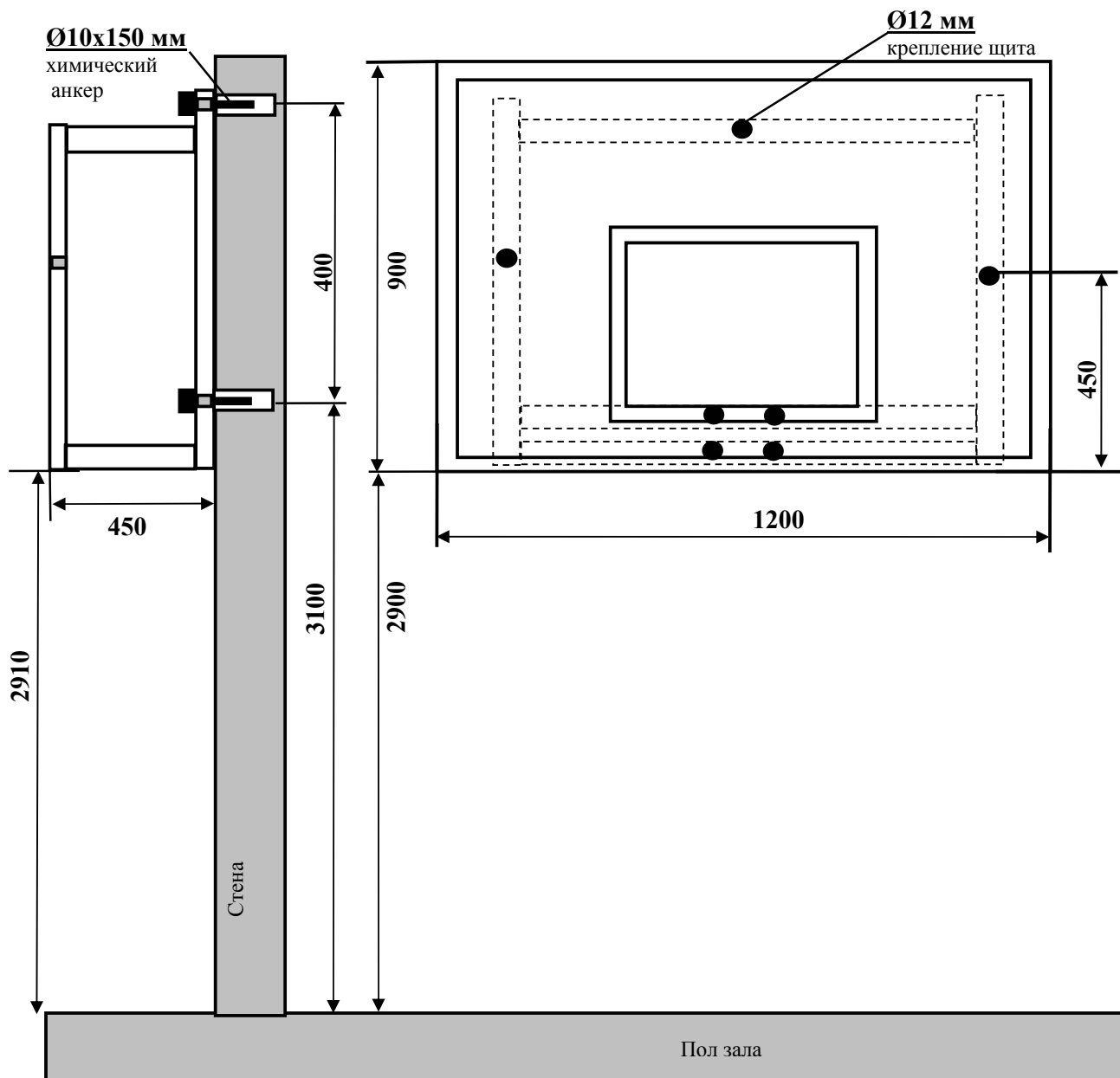
Схема монтажа баскетбольного щита размер 1200x900 мм и фермы «ED». Вылит фермы 400 мм.
