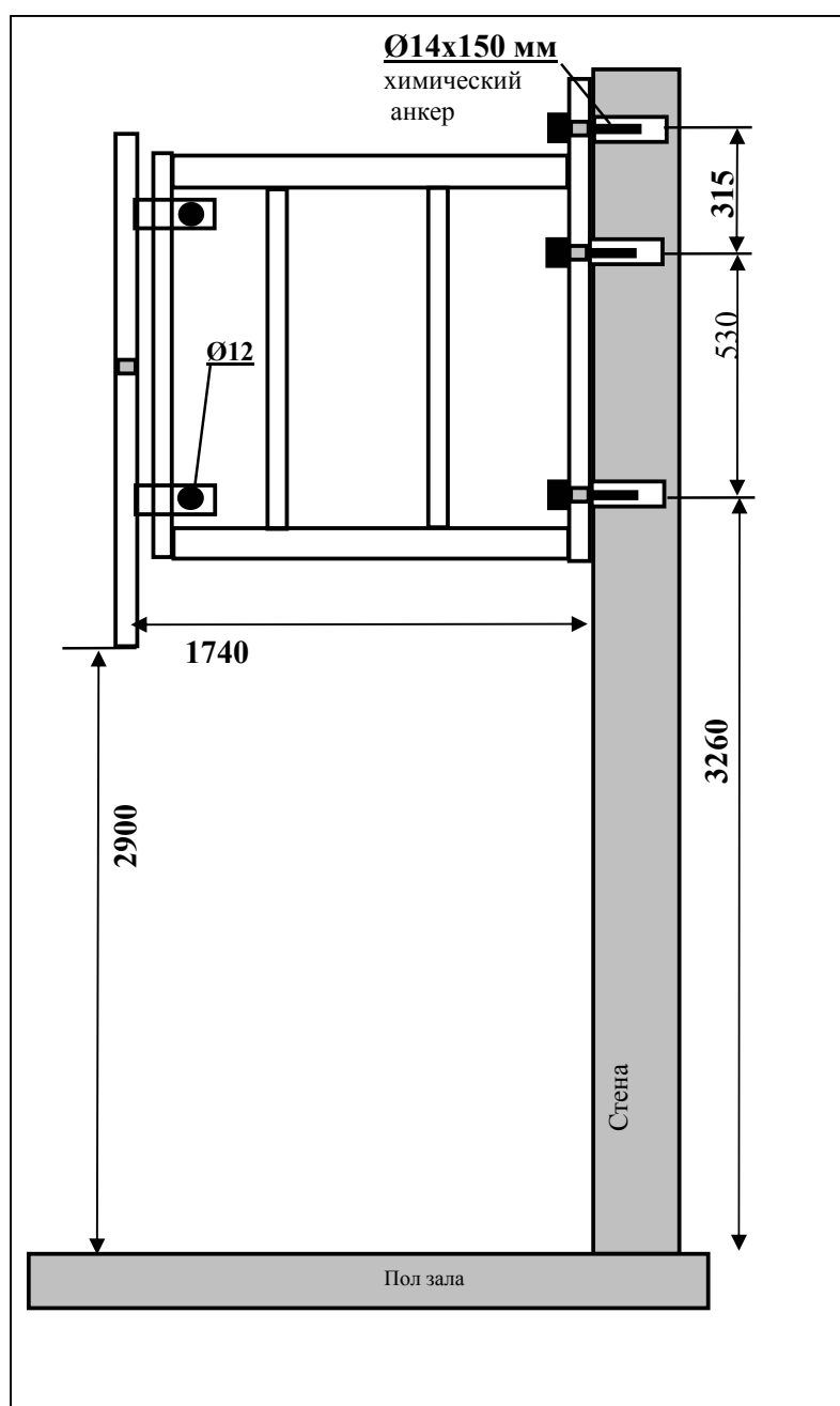
Схема монтажа баскетбольного щита размер 1800x1050 мм и фермы «ED». Вылит щита 1740 мм.
